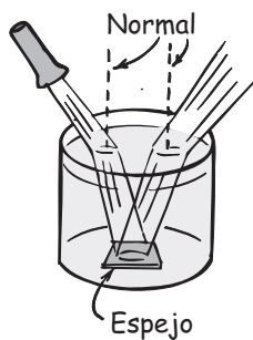
FIGURA 28.26 Cuando la luz disminuye su rapidez al pasar de un medio a otro, por ejemplo cuando pasa del aire al agua, se refracta acercándose a la normal. Cuando aumenta su rapidez al pasar de un medio a otro, como cuando pasa de agua a aire, se refracta alejándose de la normal.
