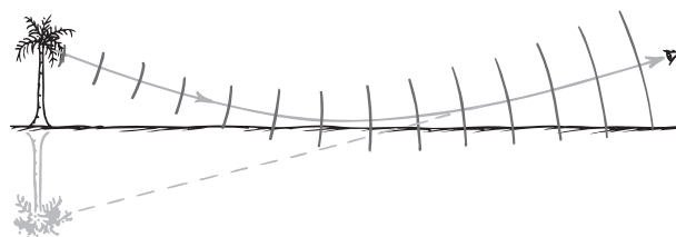
FIGURA 28.25 Una explicación ondulatoria de un espejismo. Los frentes de onda de la luz se propagan con más rapidez en el aire caliente cerca del suelo, y se curvan hacia arriba.
