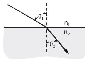
FIGURA 28.26 Cuando la luz disminuye su rapidez al pasar de un medio a otro, por ejemplo cuando pasa del aire al agua, se refracta acercándose a la normal. Cuando aumenta su rapidez al pasar de un medio a otro, como cuando pasa de agua a aire, se refracta alejándose de la normal.
